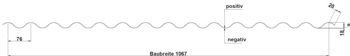
Einbausituation Wand Baubreite 1067mm
