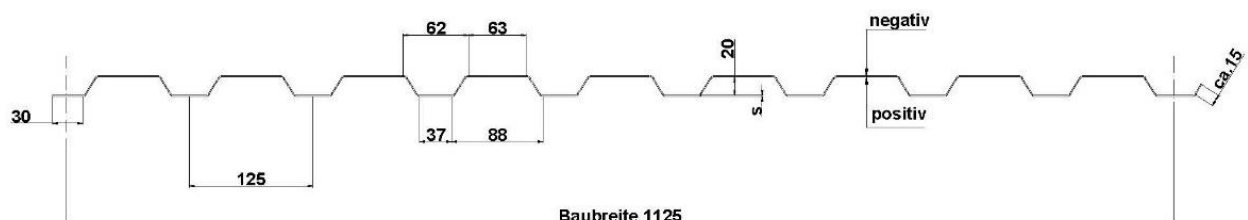
Einbausituation Wand
