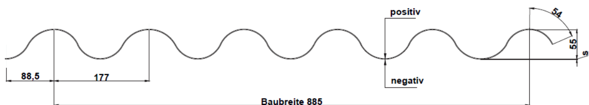
Einbausituation Dach & Wand Baubreite 885mm
