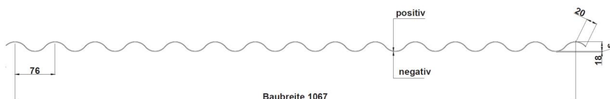
Einbausituation Wand Baubreite 1067mm
