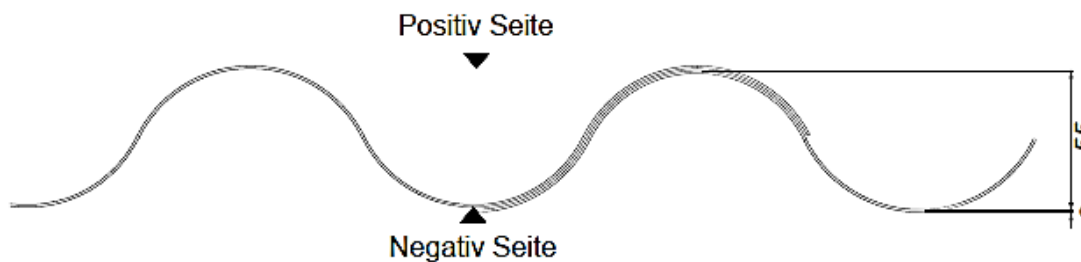
Einbausituation Dach & Wand Baubreite 885mm
