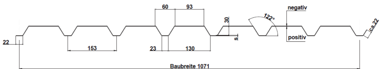
Einbausituation Dach
